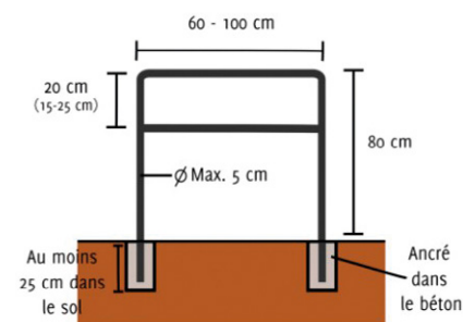
Dimensions standards d'un dispositif U renversé
